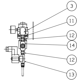
A-A SECTION
