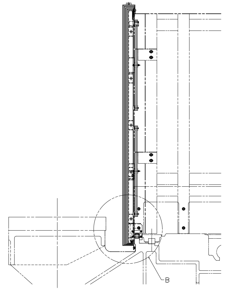
A-A SECTION
